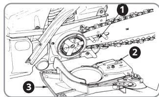
1. Orificiu 2. Știft de tensionare 3. Capac lanț
