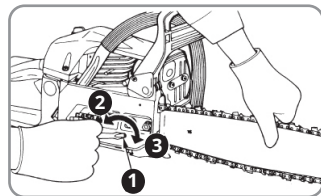
1. Șurub de tensionare 2. Slăbire 3. Strângere
