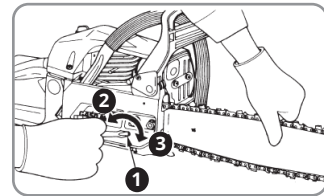
1. Spanschraube 2. Lösen 3. Anziehen
