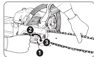
1. Spannschraube 2. Lösen 3. Anziehen
