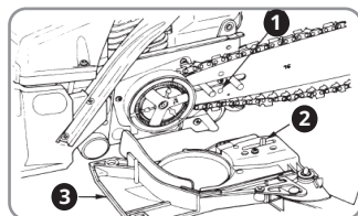
1. Loch 2. Spannstift 3. Kettenabdeckung
