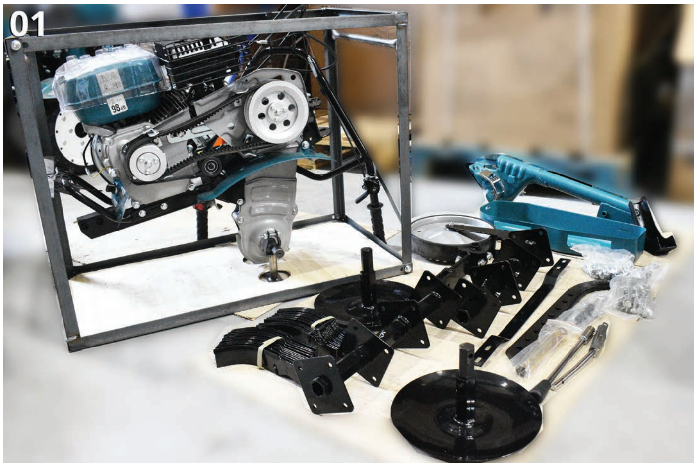
Fig. 1. Privire de ansamblu asupra cultivatorului pe benzină KS 7HP-950A în timpul pregătirii pentru asamblare.
