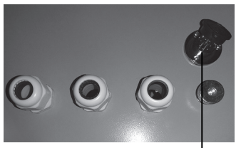
8-poliger ATS-Ausgang an der ATS-Einheit
